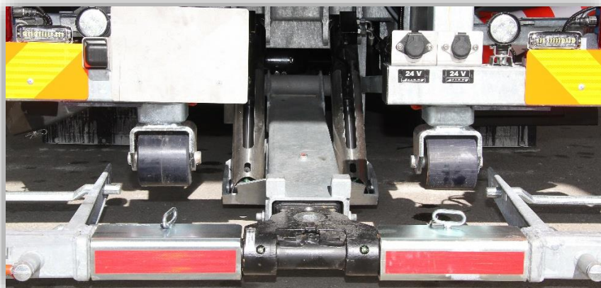
BEQUILLES REGLABLES SUR ROULETTES / REAR STABILIZERS WITH WHEELS
