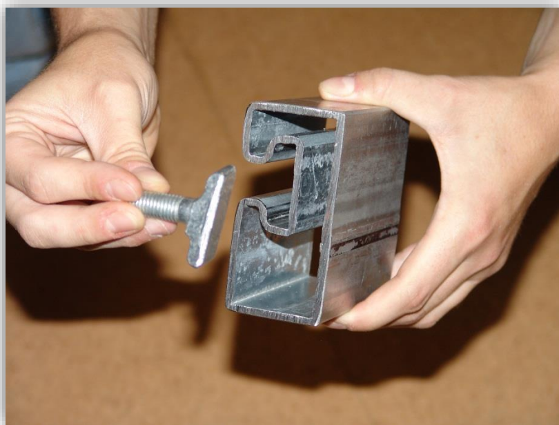
FAUX CHASSIS GALETTE EN 1 PIECE AVEC FEUILLURE PERMETTANT UNE FIXATION TOUTES POSITIONS ONE PIECE ROLL COLD SUBFRAME WITH A GROOVE ALLOWING AN EASY POSITIONING
